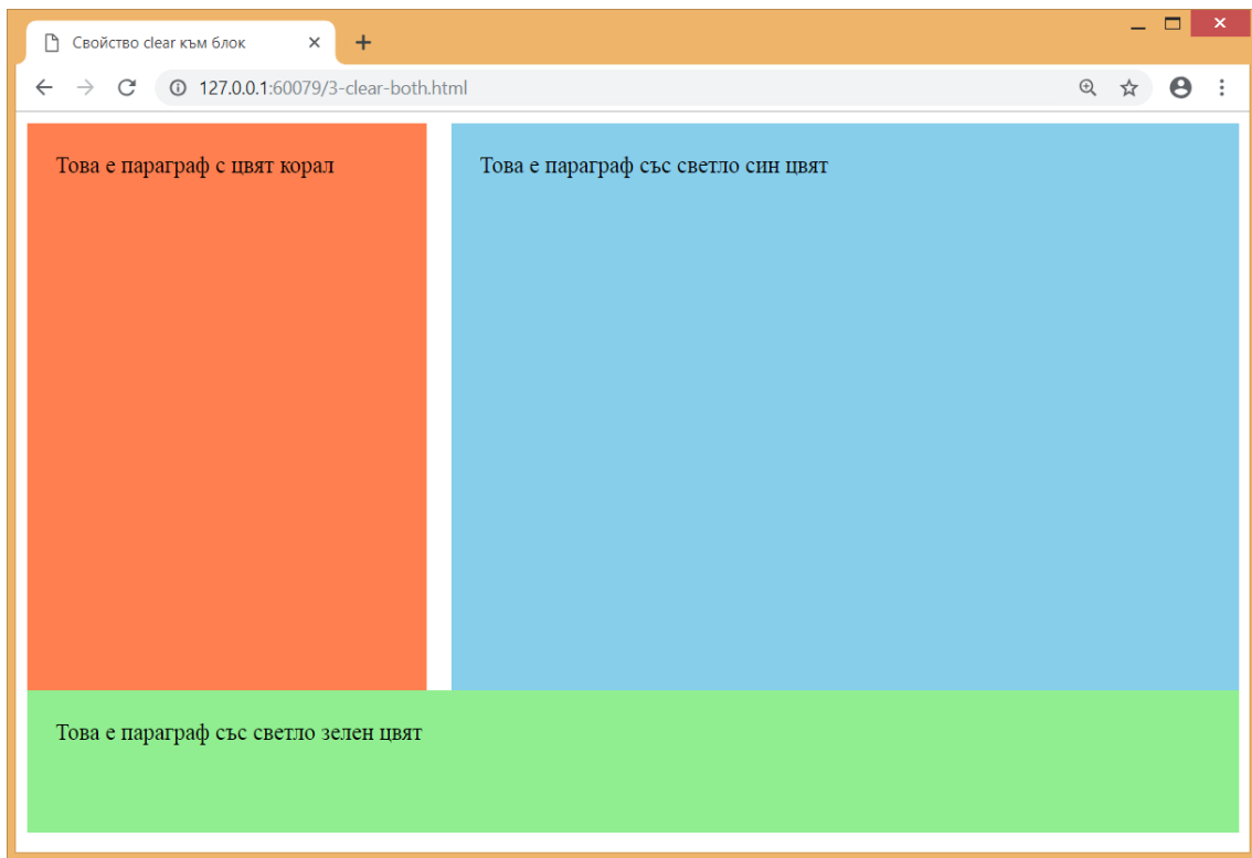
Фиг.4 Изчистване на ляво и дясно подравняване със свойство clear към блок green
